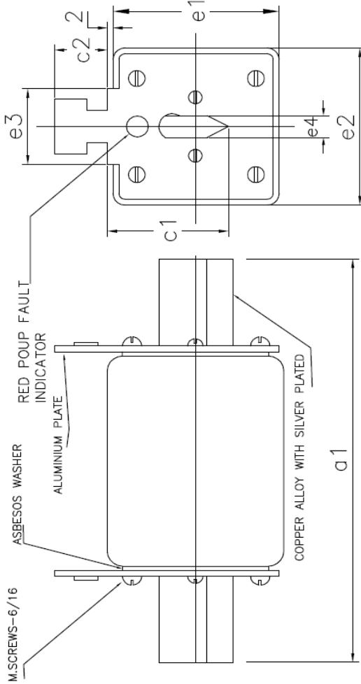
H.R.C. FUSE LINK 160 AMPS SS-01
